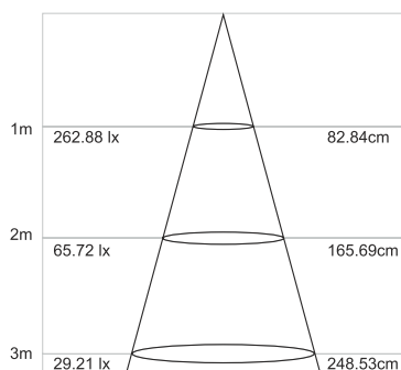
Apšvietos kreivė
